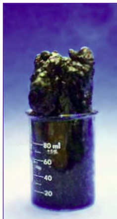
47-rasm. Sulfat kislotaning yog'ochga ta'siri.
