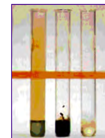
46-rasm. Mis va boshqa ba'zi metallarning turli kislotalar bilan ta'sirlashuvi.
