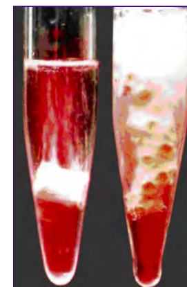
53-rasm. Xlorid kislotaning bo'rga ta'siri.
