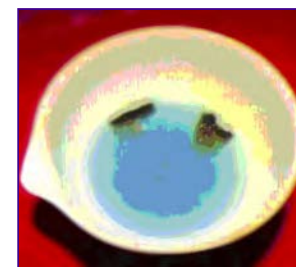
46-rasm. Mis va boshqa ba'zi metallarning turli kislotalar bilan ta'sirlashuvi.
