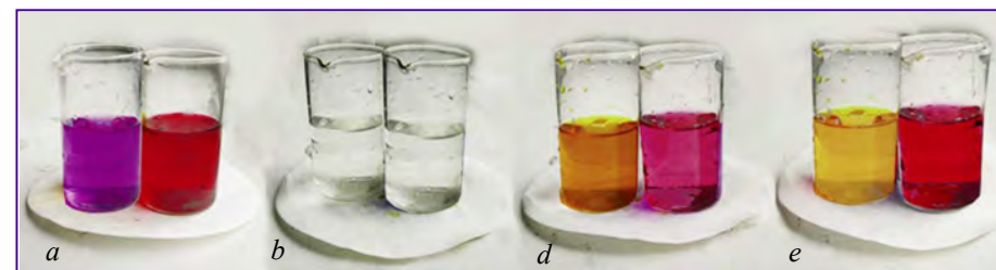
27-rasm. Kislotalar eritmalarining indikatorlarga ta'siri:
