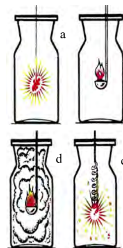
22-rasm. Kislorodning kimyoviy xossalari. Ko'miri (a), oltin-gugurt (b), fosfor (d) va temirni (e) kislorodda yonishi.
