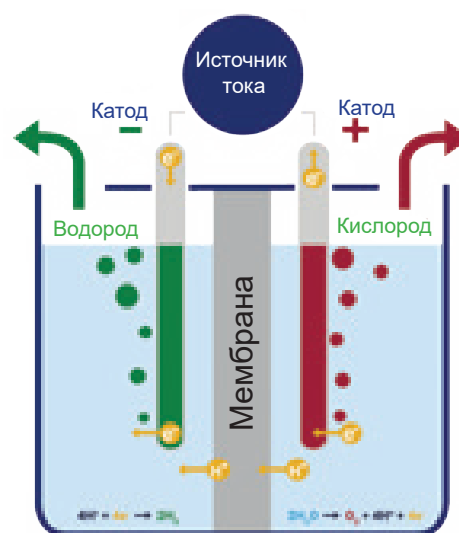
Получение кислорода из воды
