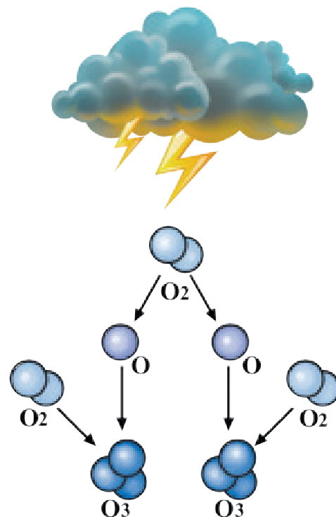
Образование озона из кислорода в природе
