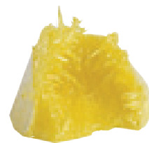
Моноклинная сера
