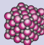
Натрий хлор в хлориде натрия
