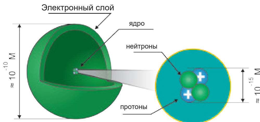
Атом гелия. Состоит из 2 протонов, 2 нейтронов, 2 электронов.
