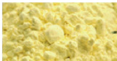
Ромбическая сера
