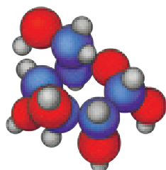
Молекула глюкозы
