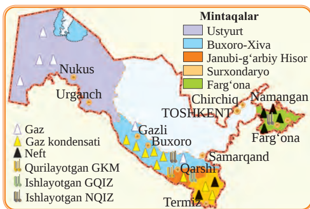
20-rasm. Neft-gazli mintaqalar.
