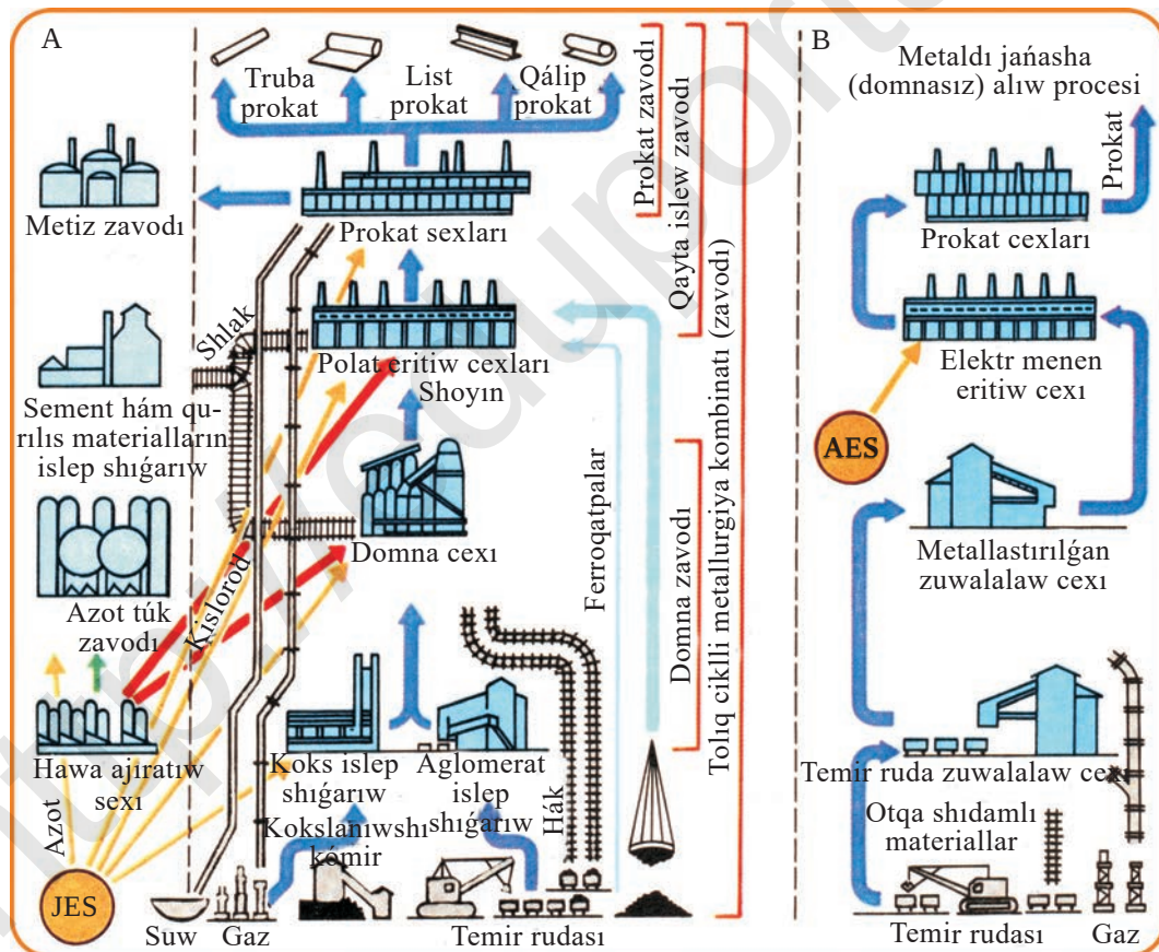
35-súwret. Metallurgiya kombinatındaǵı cexlar sxeması.
