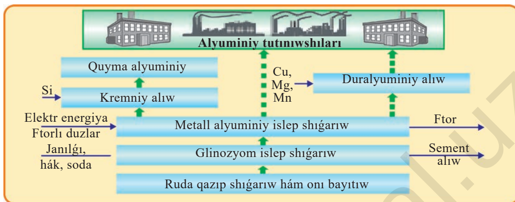
38-súwret. Alyuminiy islep shıǵarıw.
