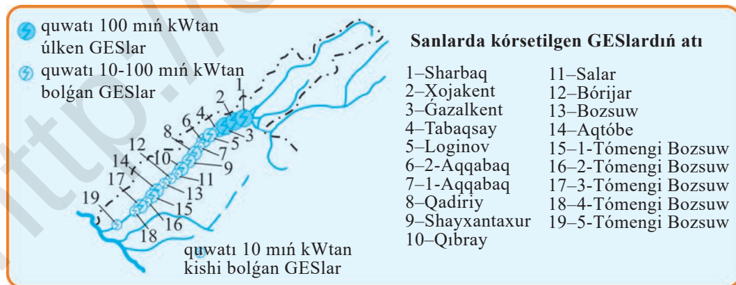
31-súwret. Chirchiq-Bozsuw gidroenergetika kaskadı.
