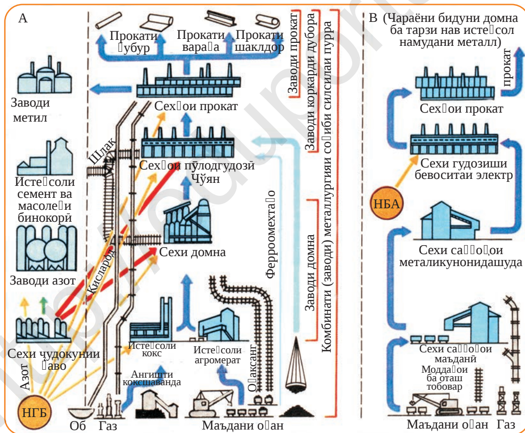
Расми 35. Схематҳои комбинати металлургӣ.
