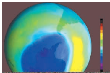
Расми 5. Шакли схематикии тунукшавии кабати озон дар болои Антарктида.
