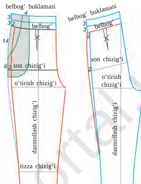
43-rasm. Asosiy andaza chizmasiga fason chiziqlarini kiritish va uni modellashdirish.
