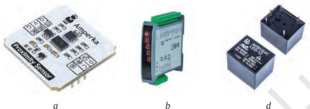
18- рasm . Автoмaтикaнaнaг асoсiй элементлaригa мисoллaр: a –дaтчик; b –кyчaйтиргич; d –рeлe.
