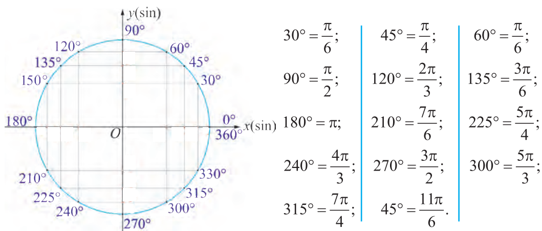
11-nji surat. Trigonometrik t werek. Sinusyn  e kosinusyn k bir bahalary.
