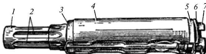
99-rasm. Gaz trubkasi stvol qoplamasi bilan birgalikda: 1—gaz trubkasi; 2—gaz porsheni uchun yoʻnaltiruvchi qovurgʻalar; 3—oldindagi biriktirgich; 4—stvol usti qoplamasi; 5—ortki biriktirgich; 6—boʻrtma; 7—yassi prujina.
