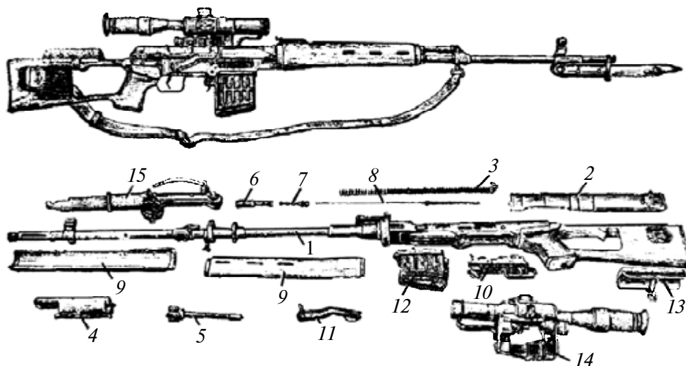
119-rasm. SDVning umumiy ko'rinishi, asosiy qism va mexanizmlari:
