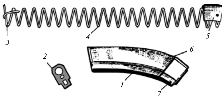
102-rasm. Magazin: 1—korpus; 2—qopqoq; 3—mahkamlovchi planka; 4—prujina; 5—yuboruvchi; 6—tayanch bo'rtmasi; 7—ilgich.
