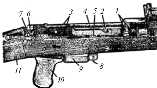
93-rasm. Stvol qutisi: 1—kesmalar; 2—qaytaruvchi boʻrtma; 3—boʻrtiqlar; 4—yoʻnaltiruvchi boʻrtma; 5—biriktirgich; 6—boʻylama oraliq; 7—koʻndalang oraliq; 8—magazin uchun moʻljallangan qistirgich; 9—tepki halqasi; 10—pistolet dastasi; 11—qoʻndoq.
