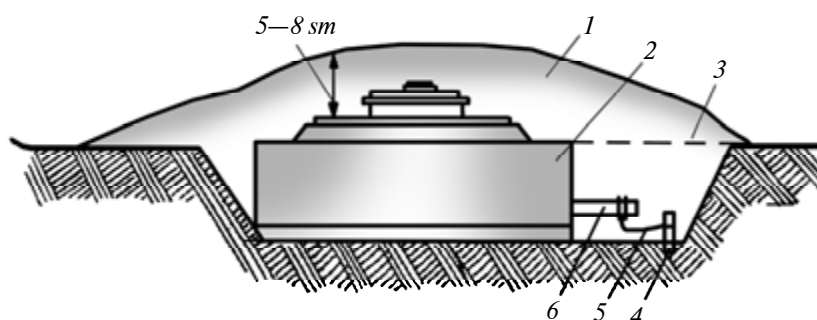
76-rasm. Tankka qarshi minaning yaydoq yerlarda oʻrnatilishi:
