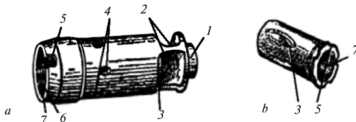
92-rasm. Ogʻiz tormozi — olov soʻndirgich (a) va kompensator (b): 1—uchki qismi; 2—tuynuklari; 3—yorma; 4—soʻndiruvchi tirqishlar; 5—biriktirgich uchun kesma; 6—aylanasiga bukilgan qismi; 7—ichki rezba.
