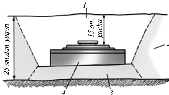
80-rasm. Qish (qor yogʻgan) sharoitda tankka qarshi minaning oʻrnatilishi: 1—niqoblovchi qor; 2—qor; 3—zichlangan qor; 4—mina.
