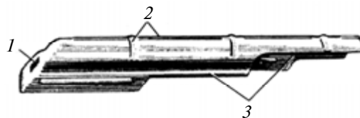
94-rasm. Stvol qutisining qopqog'i: 1—yoriq; 2—qattiq qirrasi; 3—pog'onali kesim.
