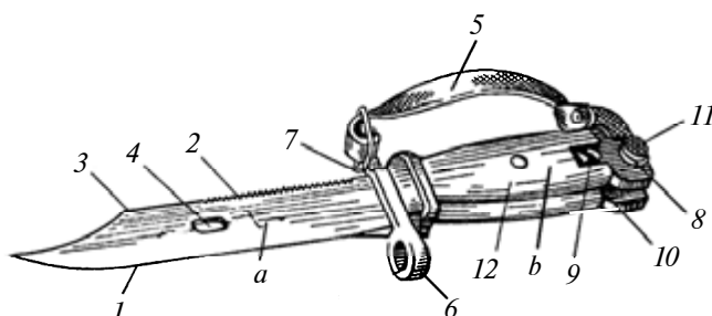
103-rasm. Nayza-pichoq: a —tigʻ; b —dasta; 1—kesuvchi qirra; 2—arra; 3—charxlangan uchi; 4—teshik; 5—kamar; 6—halqa; 7—kamar uchun ilgich; 8—dastaning metall qismi; 9—qoʻshuvchi vint; 10—boʻylama kesma; 11—tortqi; 12—sop.
