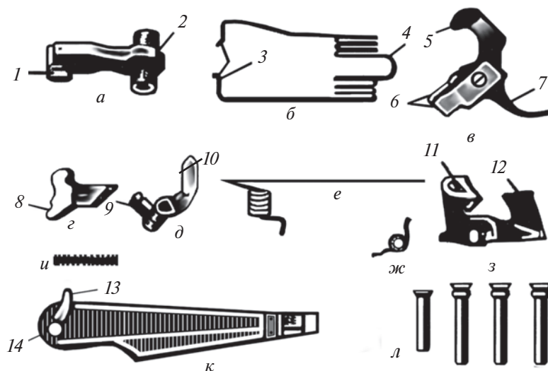
Расми 100. Қисмҳои механизми зарбадиҳанда:
