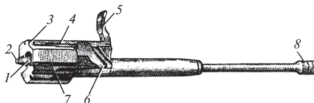
Расми 96. Рамаи затвор, яқоя бо поршени газ:
