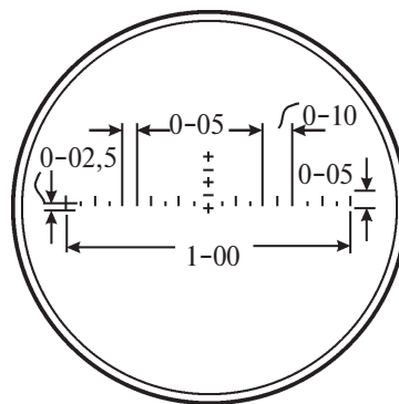
Расми 71. Намуди дурбини кунҷченкунак.
