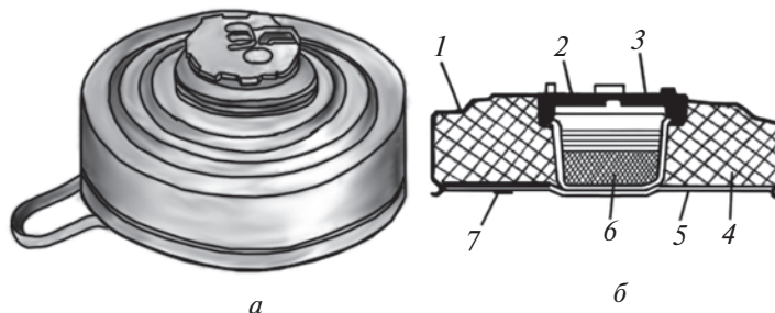
Расми 77. Минаи зиддитанкии ТМ-62 М:
