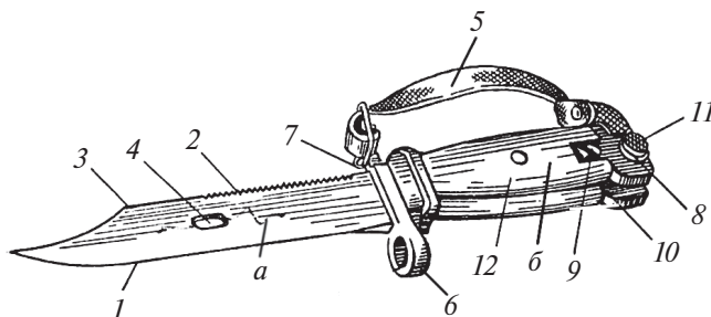
Расми 103. Найза-корд: a —теғ; б —даста; 1—қирраи бурранда; 2—арра; 3—нўғи чархшуда; 4—сўроҳи; 5—камар; 6—ҳалқа; 7—чангак барои камар; 8—қисми метали даста; 9—винти пайвасти; 10—буриш; 11—кашиш; 12—соп.
