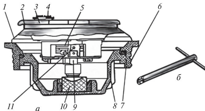
Расми 78. Тарконандаи МВСН-62:
