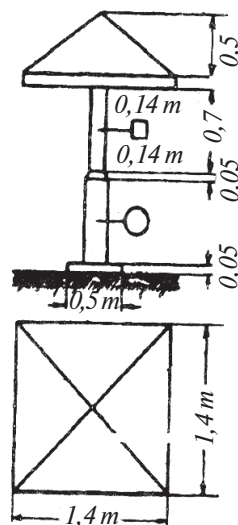
Нақшаи боми дидбони посбон.
