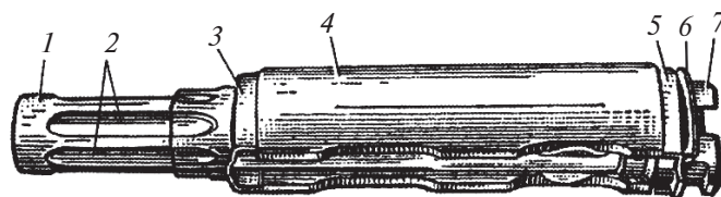
Расми 99. Трубкаи газ яқоя бо ғилофи мил: 1—трубкаи газ; 2—қабур-ғаҳои самтбахш барои поршени газ; 3—пайваस्तкунандаи пеш; 4—ғилофи болои мил; 5—пайваस्तкунандаи ақиб; 6—тобдиҳанда; 7—пружинаи паҳн.
