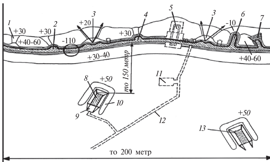
Расми 73. Сексияи хандақ: 1—майдои чанг; 2—гузаргоҳҳо ба паҳлӯ; 3—қойи пулемётҳо; 4—қойи оташфишони; 5—истеҳкоми болопӯшида; 6—қойи гранатомёт; 7—майдои чангии болопӯшида; 8—қой барои БМП дар позитсияи асосии оташфишони; 9—аппарел; 10—тўдаи хок; 11—қойи зарурат; 12—роҳҳои алоқа; 13—қой барои БМП дар вазъияти аз захира оташ кушодан.
