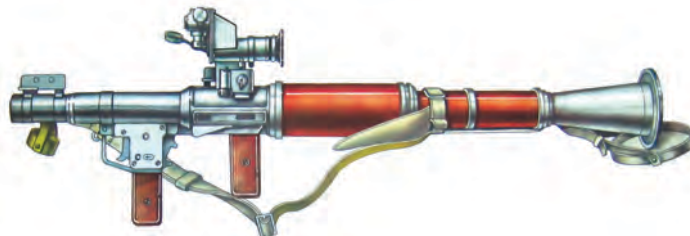
Расми 121. РПГ-7D гранатомёти дастии зиддитанки.
