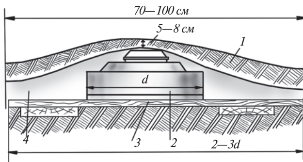
Расми 79. Гузоштани минаи зиддитанкӣ дар замини мулоим (зах) yerda: 1—қабати ниқоби; 2—мина; 3—зермони тахтагӣ; 4—бо хок доштан.
