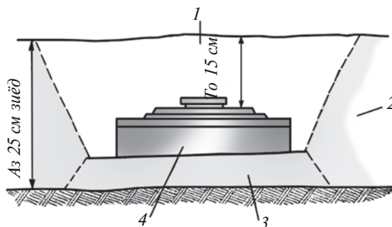
Расми 80. Гузоштани минаи зиддитанки дар зимистон (барф): 1—барфи ниқоби; 2—барф; 3—барфи зичшуда; 4—мина.
