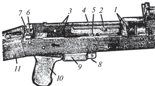
Расми 93. Қуттии мил: 1—буришҳо; 2—бозгардон; 3—барҷастаҳо; 4—барҷастаи самтноккунанда; 5—пайвасткунанда; 6—фосилаи яксара; 7—фосилаи буришӣ; 8—исканҷаи магазин; 9—ҳалқаи теладиҳанда; 10—дастаи пистолет; 11—қундоқ
