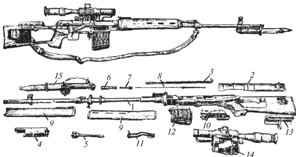
Расми 119. Намуди умумӣ, қисмҳои асосӣ ва механизмҳои СДВ:
