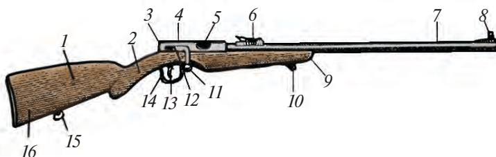
Расми 122. Милтиқи калибраш хурд (ТОЗ-8):
