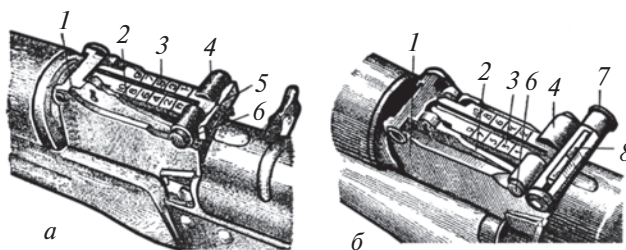
Расми 95. Ускунаи нишонгирӣ: а—барои автомат; б—барои пулемёт;
