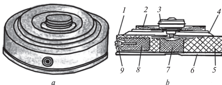
Расми 74. Намуди минаи зиддитанкии ТМ-57 бо тарконандаи MVZ-57: a —намуди умумӣ дар ҳолати нақлиётӣ; b —намуди ҳолати ҷангии мина дар бурриш: 1—корпус; 2—сипарча; 3—тарконандаи MVZ-57; 4—диафрагма (парда монеа); 5—заряд; 6—зер; 7—детонатори маркази; 8—детонатори паҳлӯ; 9—сарпӯш.
