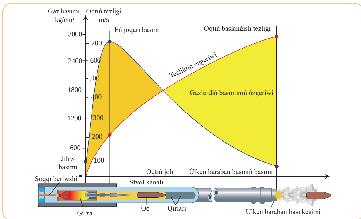
Ishki ballistika. Gazler basımınıń ózgeriwi
