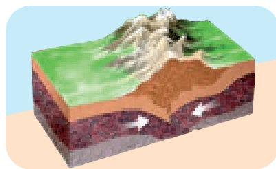
Процесс образования горы в результате движения земной коры
