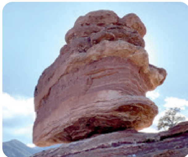
«Каменные грибы» и песчаные барханы, образованные ветром.
