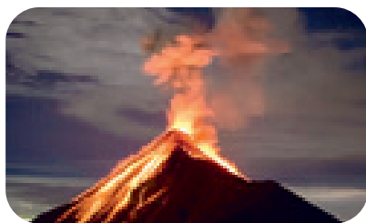
Гора, образовавшаяся в результате извержения вулкана
