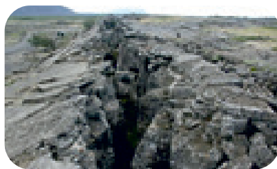
Овраг, образовавшийся в результате землетрясения
