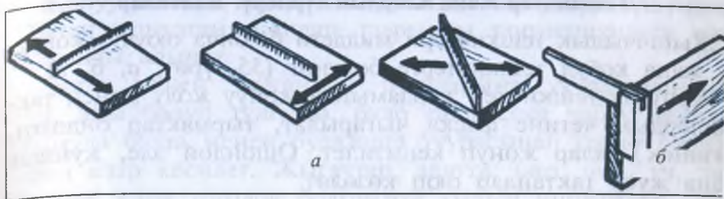
54-сүрөт. Беттердин тегиздигин сызгыч (а) же гонияда (б) текшерүү.
