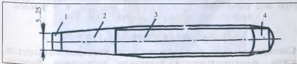
10-сүрөт. Слесардык зубилосу: 1 — мизи; 2 — ишчи бөлүгү 3 — ортоңку бөлүгү; 4 — бөркү.
