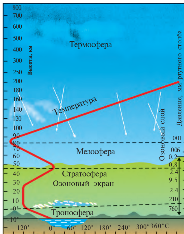
Рис. 6. Строение атмосферы
