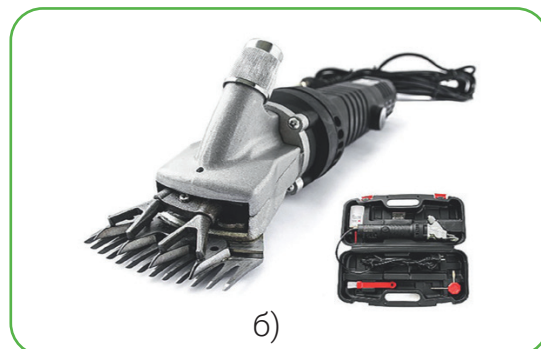
Рисунок 32. Инструменты для стрижки овечьей шерсти:
