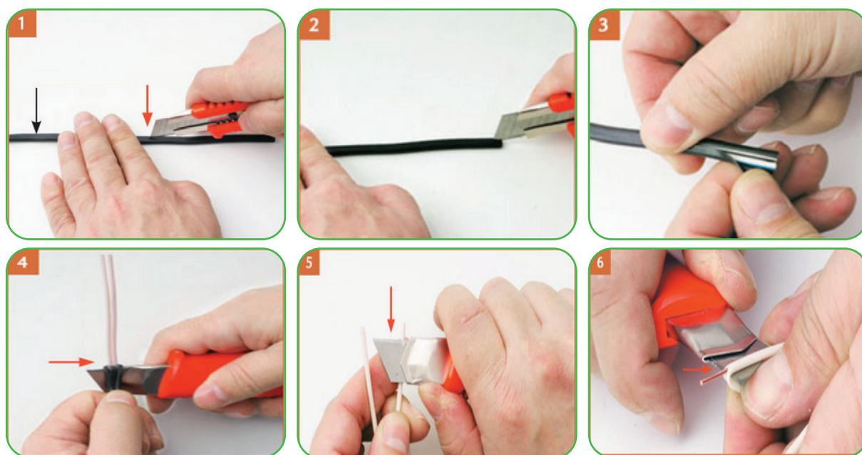
Рисунок 90. Этапы снятия изоляции электропроводов
