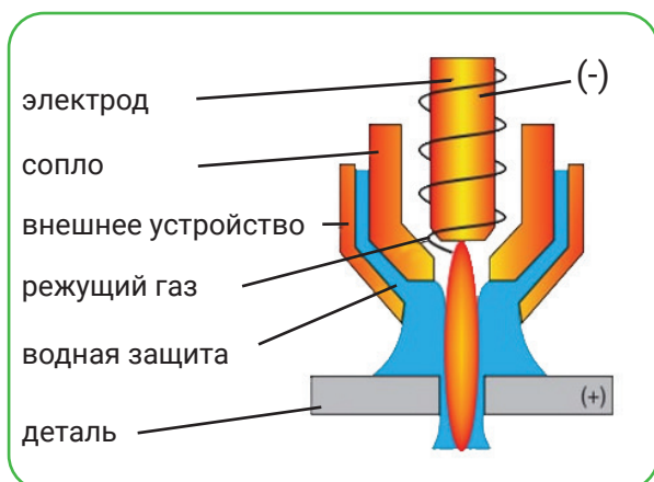
Рисунок 53. Устройство плазматрона
