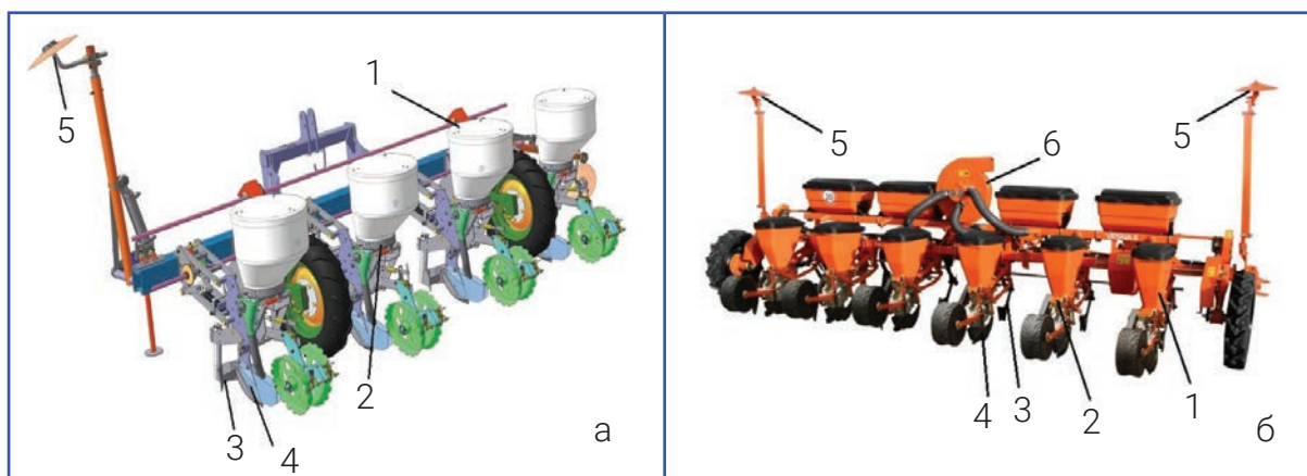
Рисунок 11. Общий вид модульной сеялки семян:
