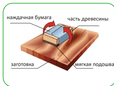
Рисунок 43. Способы закрепления наждачной бумаги
