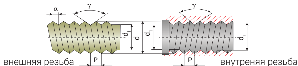
Рисунок 72. Основные элементы резьбы
