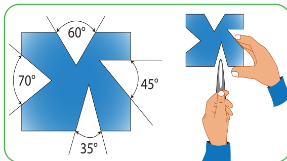
Рисунок 56. Шаблон для проверки угла заточки
