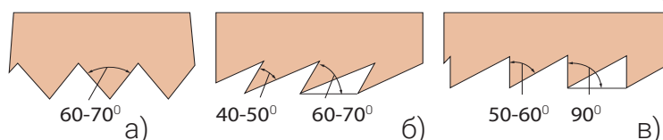
Рисунок 19. Форма зубьев пилы
