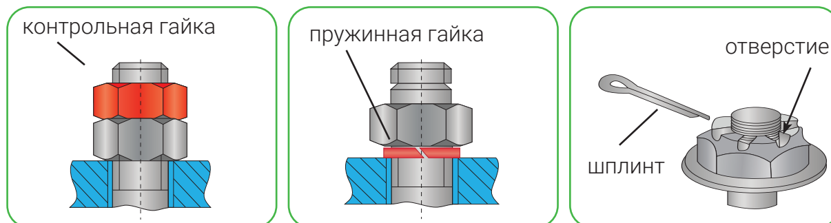
Рисунок 74. Стопорение резьбовых соединений
