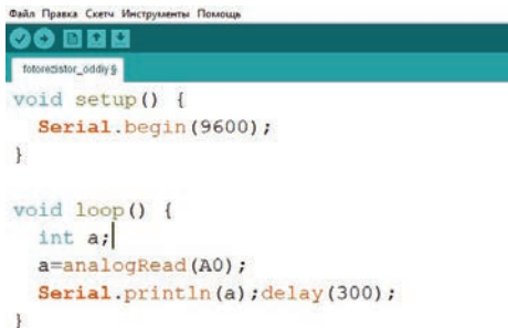
Рисунок 3. Запись программы Arduino на рабочий стол
