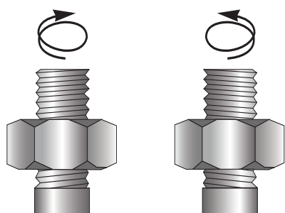
Правая резьба Левая резьба
