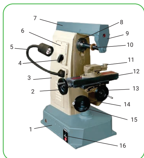
Рисунок 62. Устройство горизонтально-фрезерного станка: 1 – основание; 2 – маховик, осуществляющий продольное движение стола с помощью винтового механизма; 3 – опорная часть станка (корпус); 4 – рукоятка переключения частоты вращения шпинделя; 5 – светильник; 6 – коробка скоростей; 7 – хобот; 8 – шпиндель; 9 – подвеска; 10 – оправка установки фрезы; 11 – зубчатая рейка; 12 – стол; 13 – маховик поперечного перемещения стола; 14 – консоль; 15 – маховик для вертикального перемещения стола; 16 – кнопки управления.
