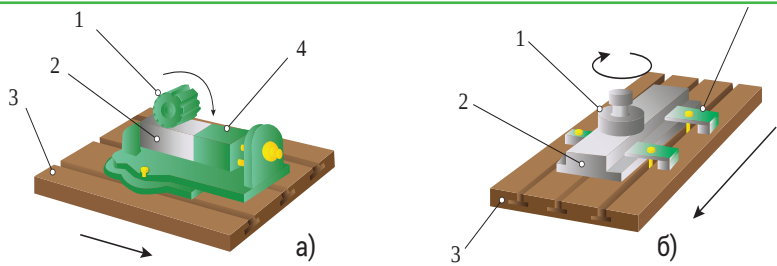
Рисунок 63. Фрезерование поверхностей: а) фрезерование цилиндрической фрезой с установкой заготовки на зубчатой рейке; б) фрезерование торцевой фрезой установленной заготовки стола, где: 1 – фреза; 2 – заготовка; 3 – стол; 4 – зубчатая рейка; 5 – зажим
