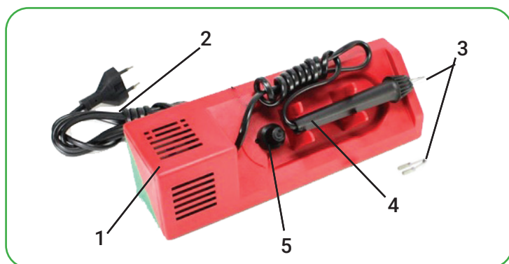
Рисунок 33. Электровыжигатель: 1 – корпус; 2 – электропровода; 3 – нагревательные наконечники; 4 – ручка, 5 – регуляторная ручка выжигателя.
