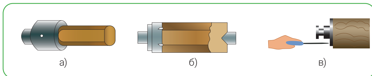
Рисунок 25. Способы закрепления заготовок на токарном станке: а) закрепление заготовки в патроне; б) закрепление заготовки в трезубце; в) закрепление заготовки в планшайбе.
