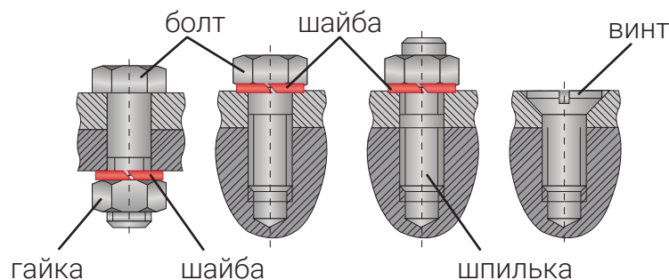
Рисунок 73. Резьбовое соединение
