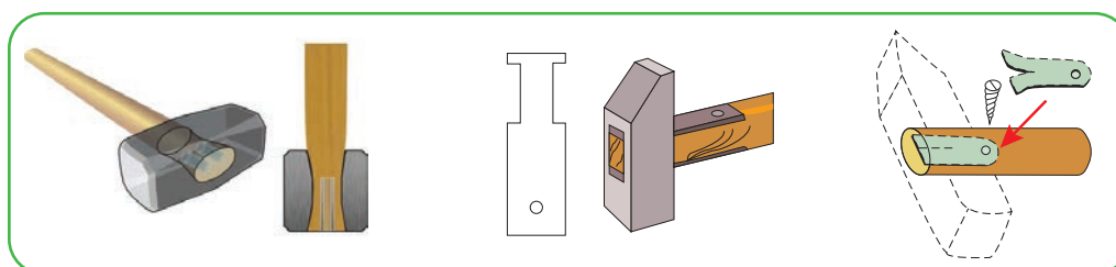
Рисунок 60. Способы крепления рукоятки молотка
