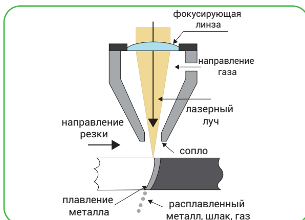
Рисунок 52. Рисунок лазерной резки листовых
