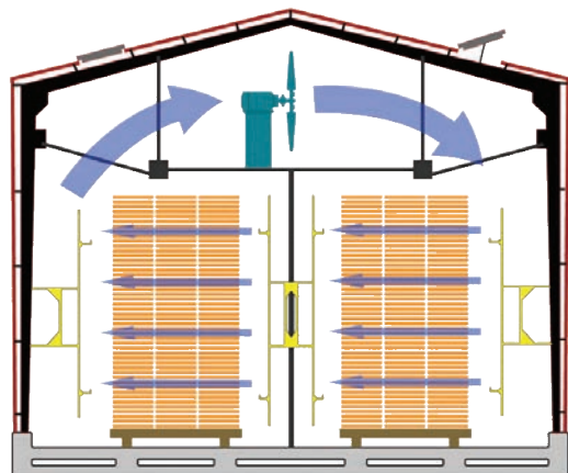
Рисунок 10. Устройство сушильной камеры
