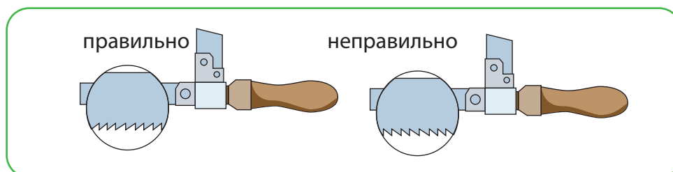
Рисунок 59. Установка зубьев полотна
